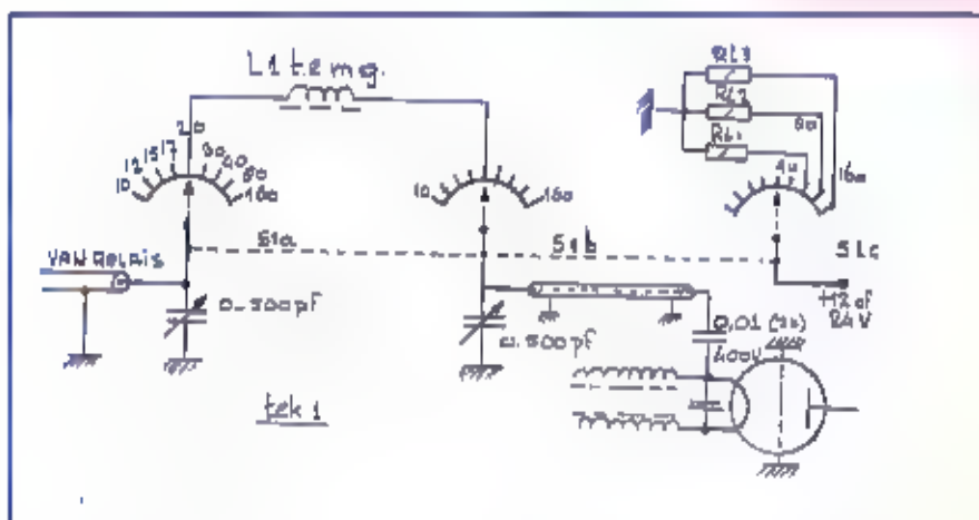
Tekening 1: het ingangsfILTER.
